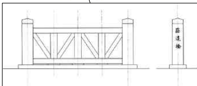
筋交橋立面図
