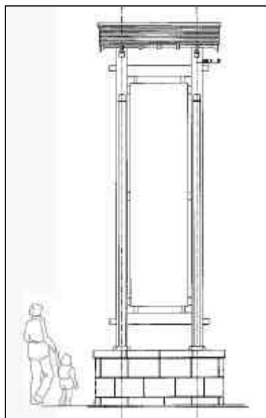
櫛比小学校前 大看板立面図
